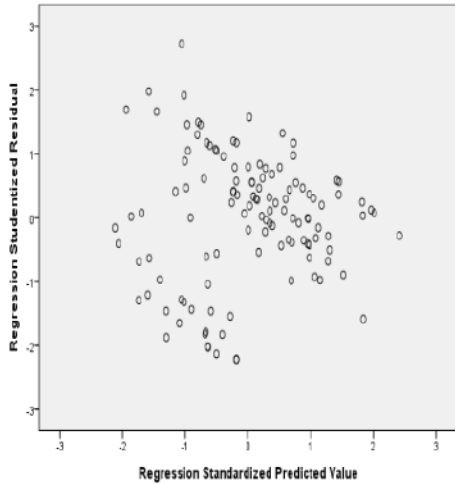
Gambar 1. Grafik hasil uji heteroskedastisitas
